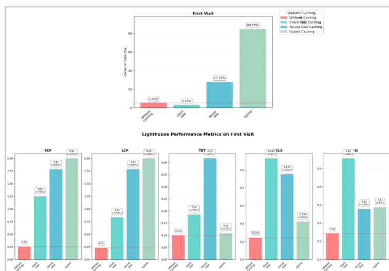
Gambar 3. Grafik Hasil Pengujian dengan Lighthouse pada First Visit
