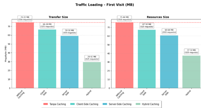
Gambar 5. Grafik Perbandingan Hasil Pengujian Traffic Loading pada First Visit
