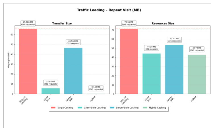
Gambar 6. Grafik Perbandingan Hasil Pengujian Traffic Loading Pada Repeat Visit
